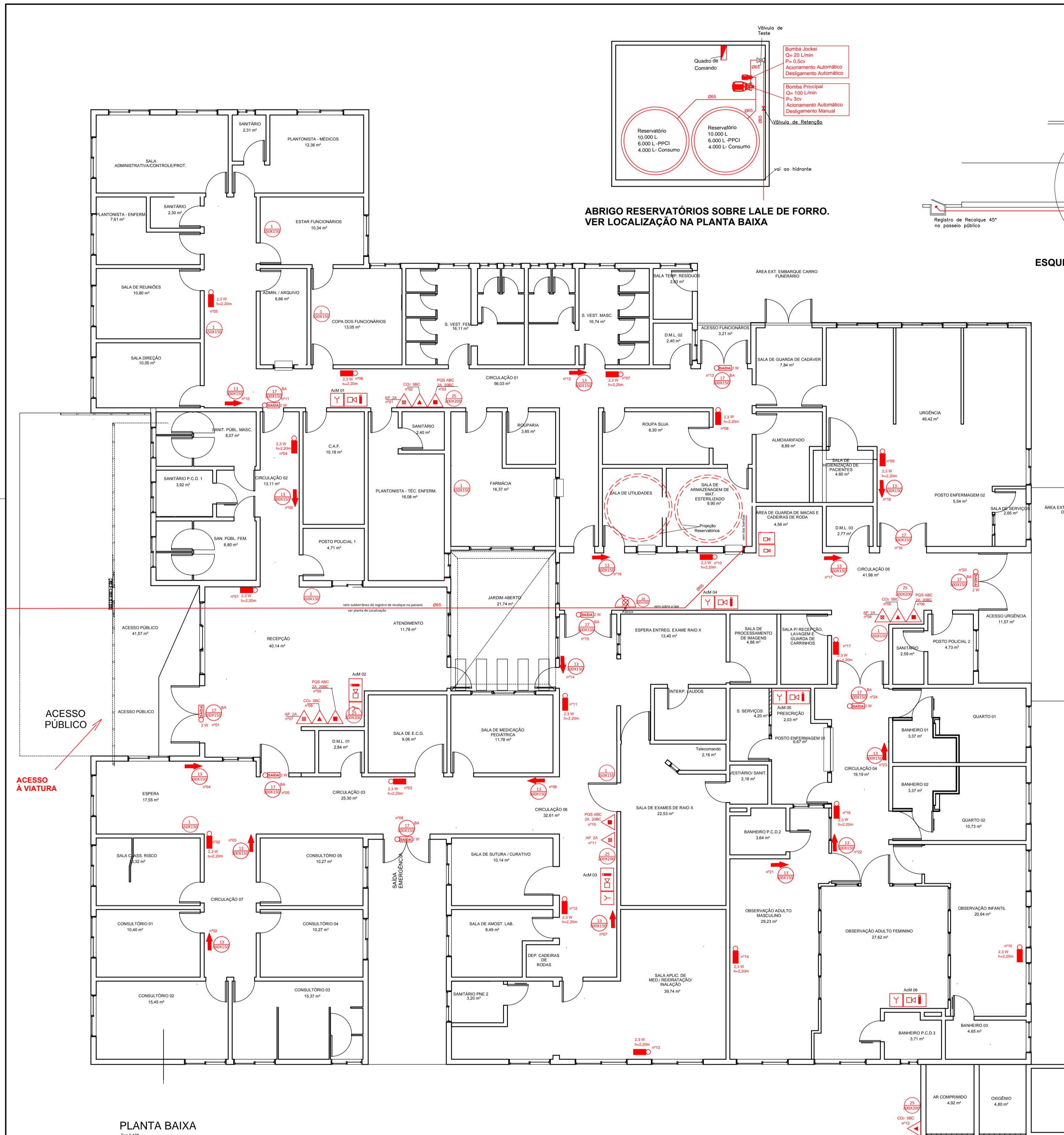
PLANTA BAIXA Ede: 1:100 H-3 - Posto de Atendimento de Urgência -450M 2 /m 2 UNIDADE DE PRONTO ATENDIMENTO - 'UPA'
