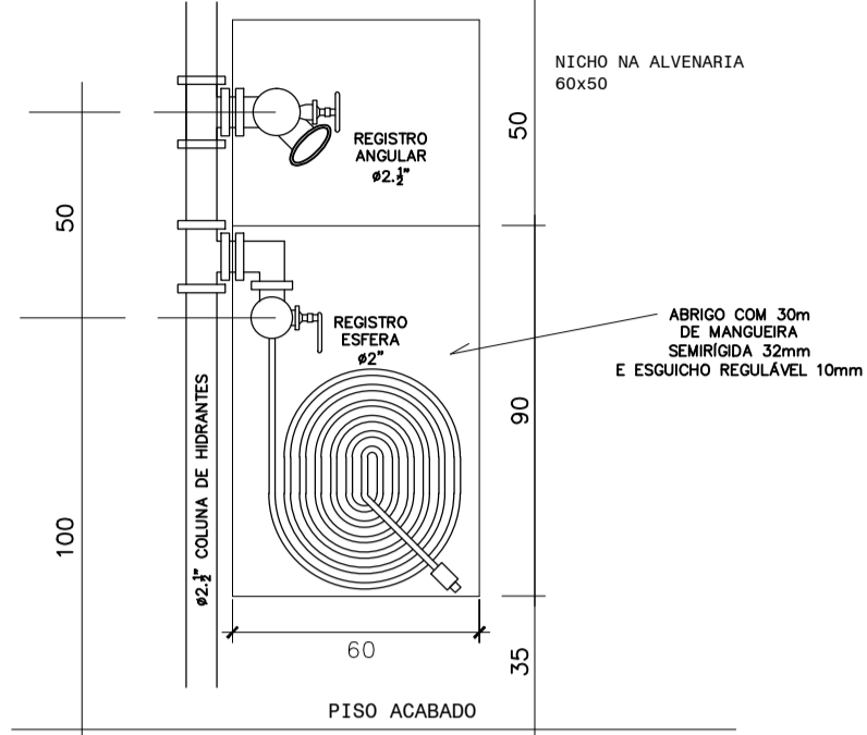
VISTA ESCALA 1/20 DETALHE CAIXA DE MANGOTINHOS
