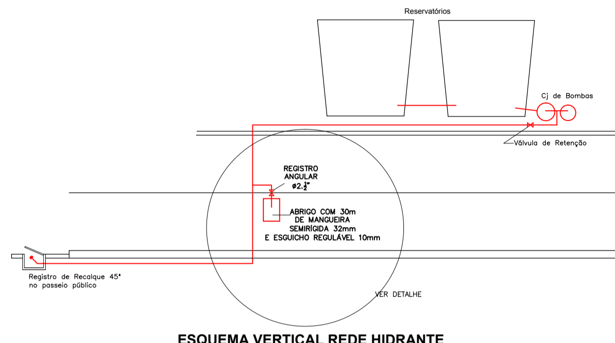
ESQUEMA VERTICAL REDE HIDRANTE
