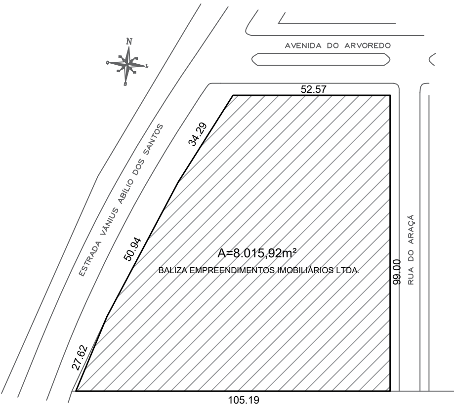
Situação Esc.: 1/1250
